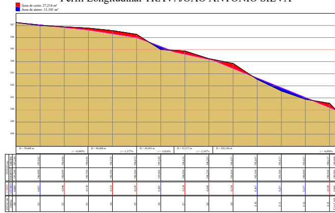
Perfil Longitudinal TRAV. JOAO ANTONIO SILVA
