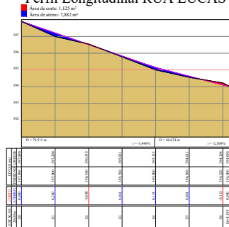
Perfil Longitudinal RUA LUCAS
