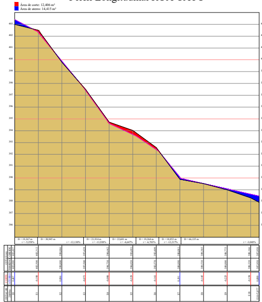
Perfil Longitudinal RUA CATU
