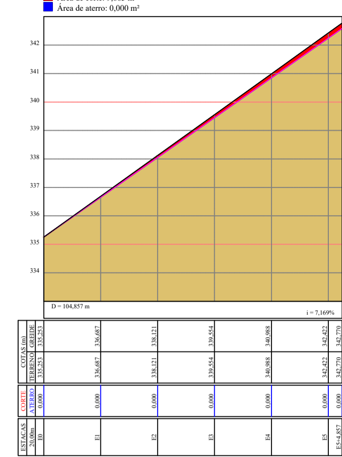
Perfil Longitudinal RUA PANORAMA
