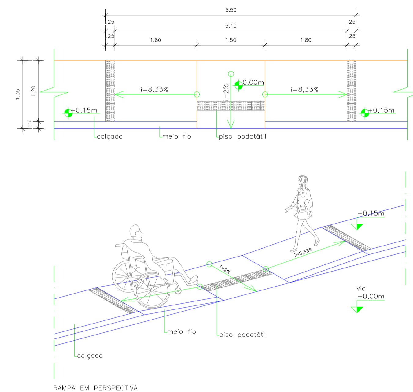
RAMPA EM PERSPECTIVA
