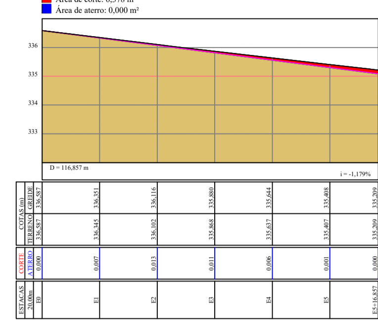
Perfil Longitudinal RUA D
