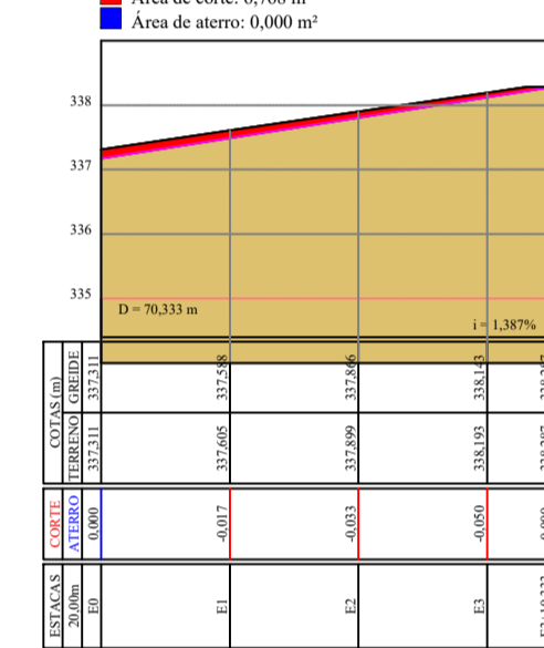
Perfil Longitudinal RUA E (TRECHO 01)
