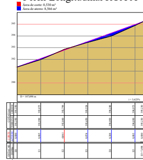
Perfil Longitudinal RUA A
