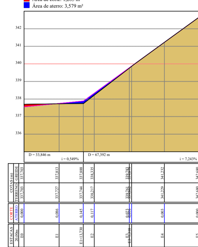
Perfil Longitudinal RUA E (TRECHO 02)
