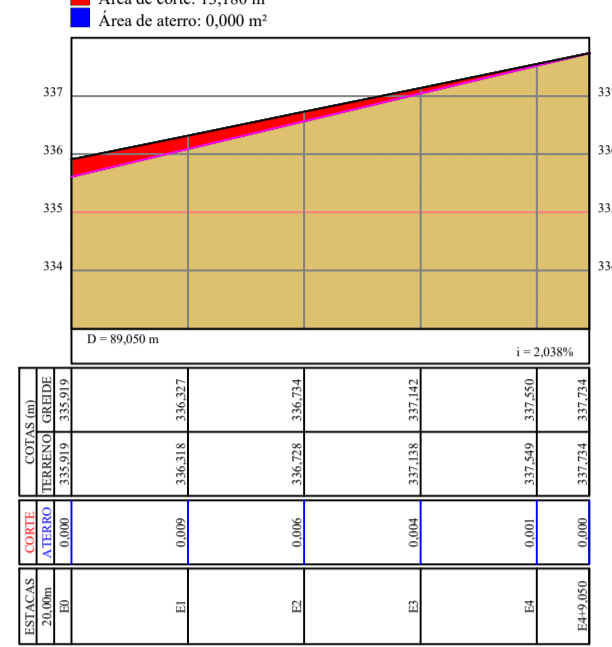
Perfil Longitudinal RUA C
