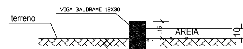
Corte A-A Sem escala
