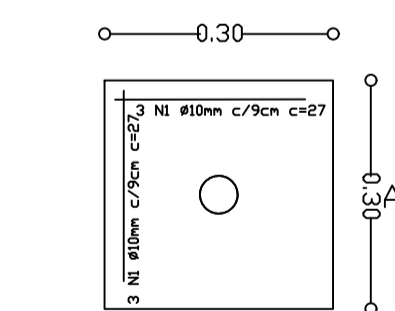
Planta baixa Sem escala
